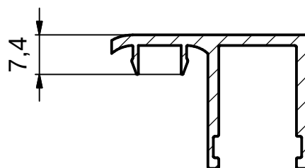
A-A ( 1 : 1 )
